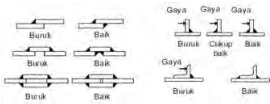
Sambungan las yang baik atau buruk berdasarkan bending momen
